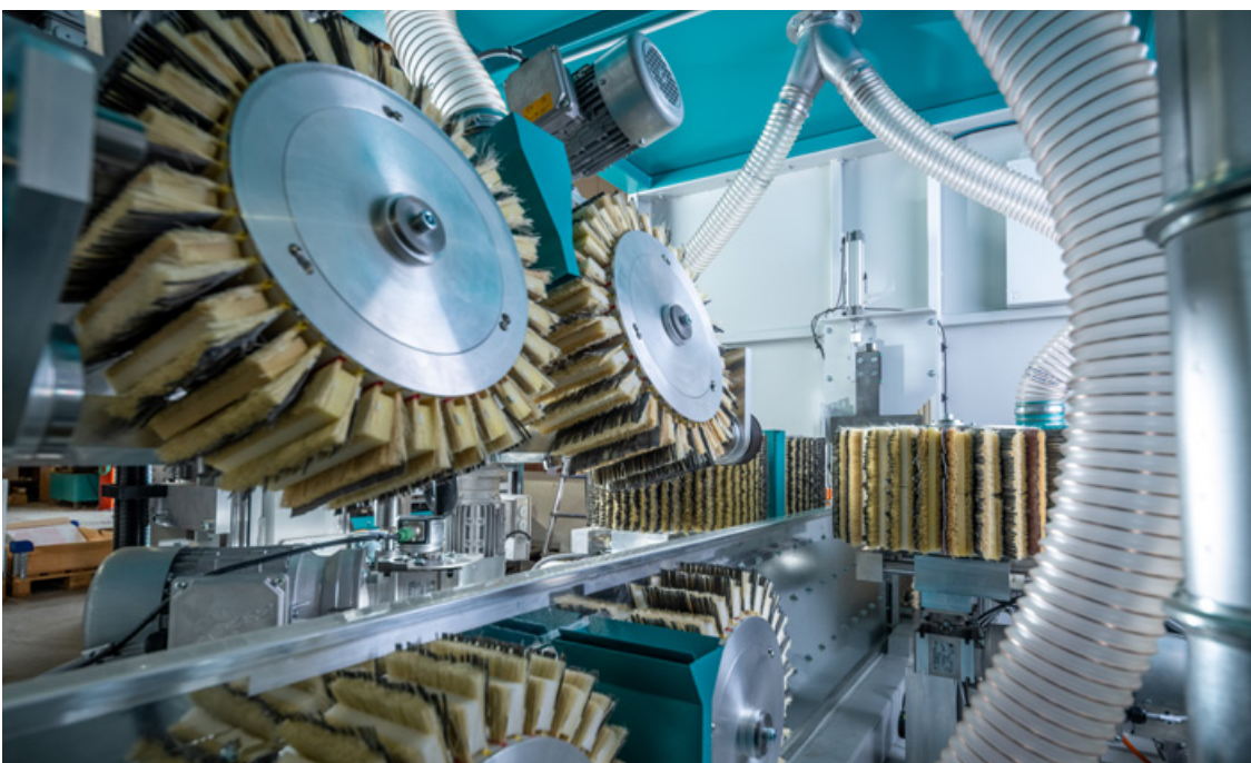
MB Flex Schleif-Werkzeuge sind in vielen Durchmessern und Längen erhältlich.
