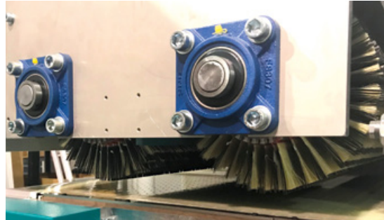
Doppelbürstenaggregat im Gleich- und Gegenlauf. Bestückung mit leicht austauschbaren Schleifsegmentbürsten
