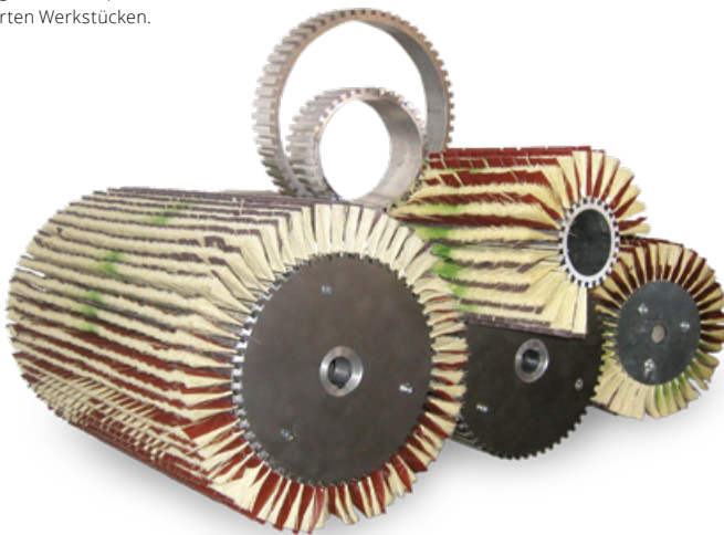
Die MB Soft Stützbürste mit Schaumstoffrücken erzielt bessere Schleifergebnisse bei profilierten Werkstücken.
